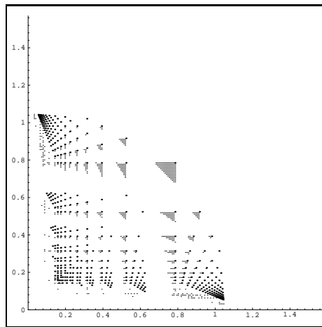
Fig. 16: Parameter set of generator (b)
