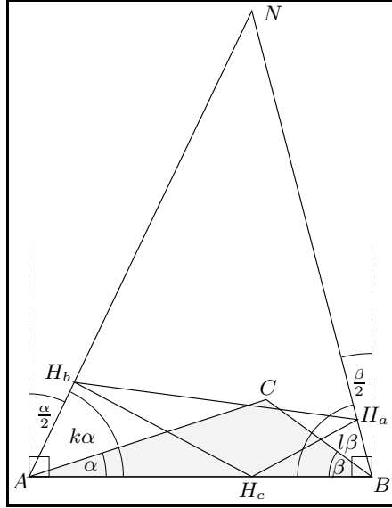
Fig. 8: Generator 132(12)^{k-1}(13)^{l-1}
