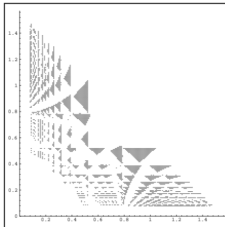
Fig. 18: Parameter set of generator (f)
