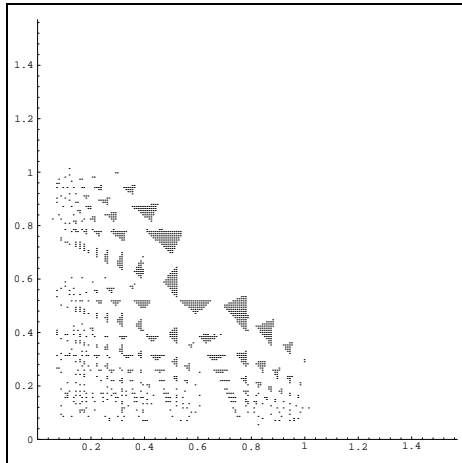
Fig. 19: Parameter set of generator (g)
