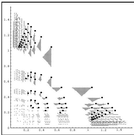
Fig. 15: Parameter set of generator (a)
