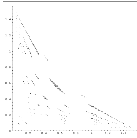
Fig. 20: Parameter set of generator (h)
