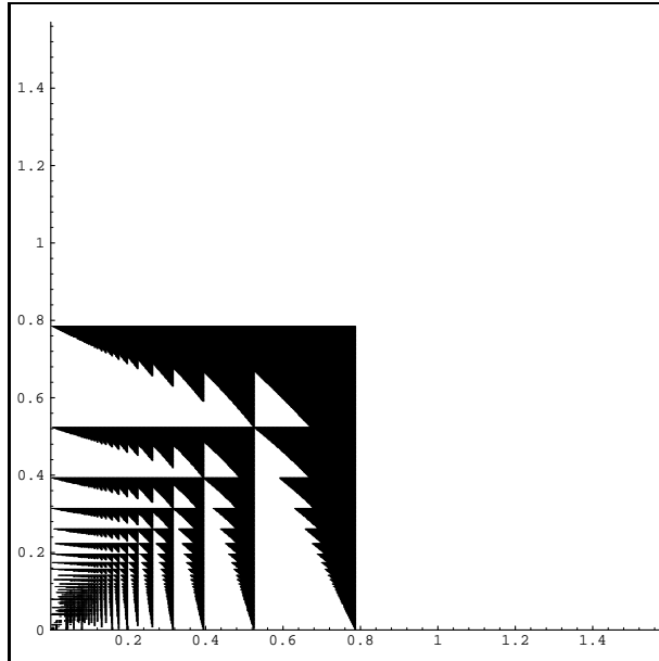
Fig. 9: Generator 132(12)^{k-1}(13)^{l-1}
