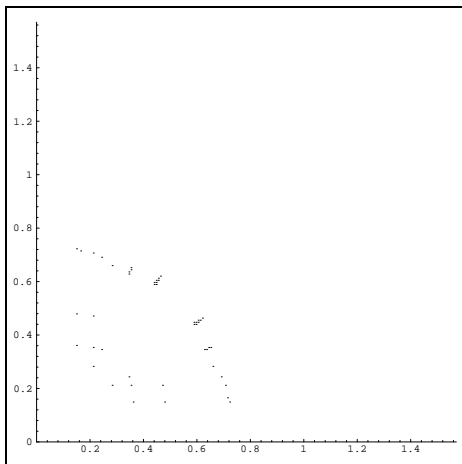
Fig. 17: Parameter set of generator (c)
